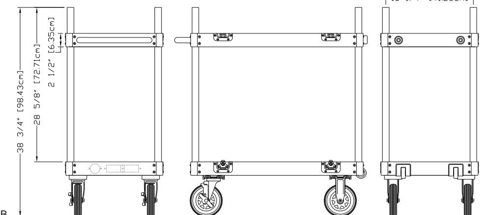
TR-06 MINI with (2) Standard AC Outlets
